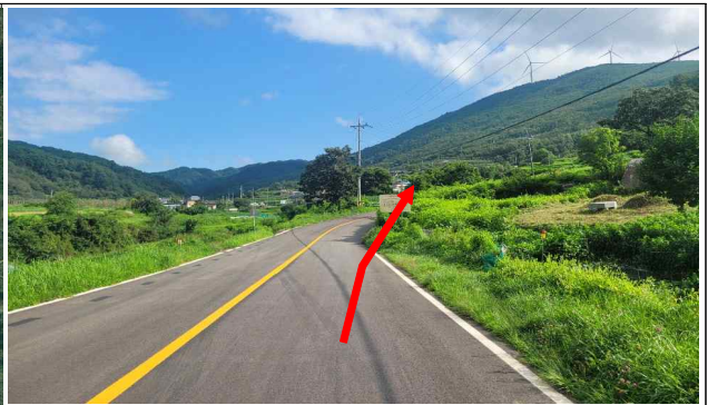
굴곡도로 선형개량
