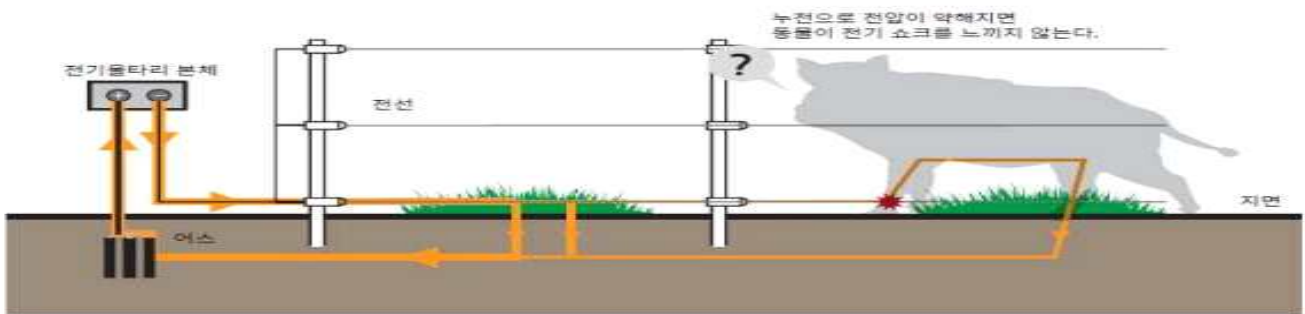
[그림 4-1] 잡초나 작물이 전선에 접촉하는 것에 의한 누전
