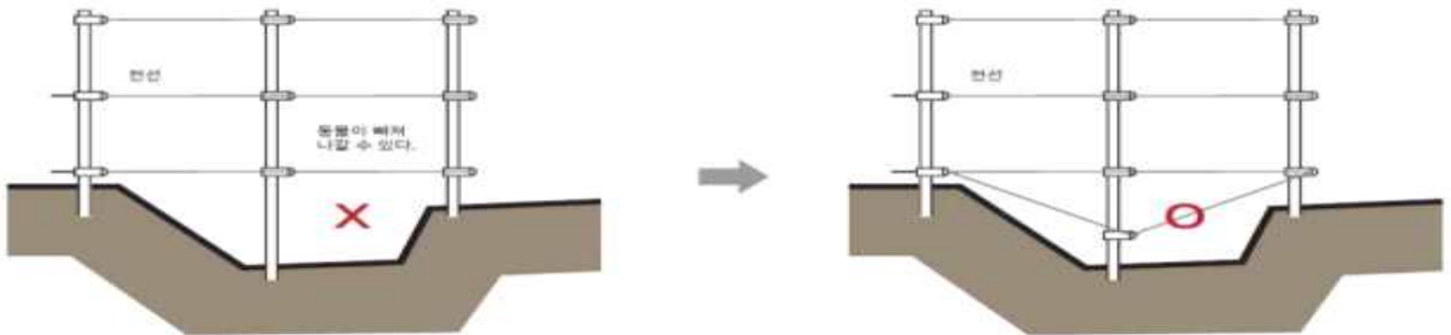
[그림 4-3] 지면이 고르지 못한 경우의 전기울타리 설치
