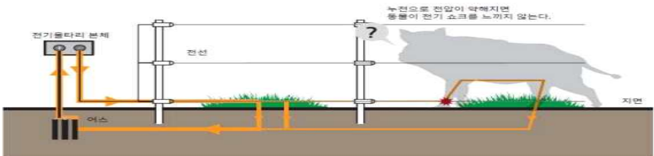
[그림 4-1] 잡초나 작물이 전선에 접촉하는 것에 의한 누전
