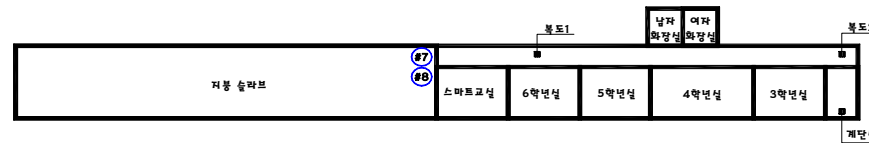
지상2층 평면도
