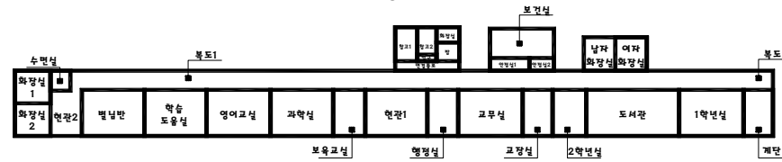
지상1층 평면도
